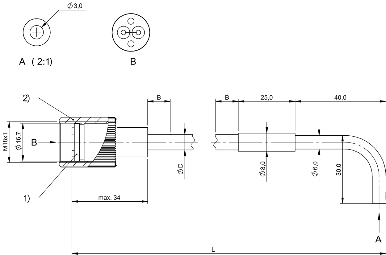
1) 墊片, 可拆式, 2) 鎖緊螺母
