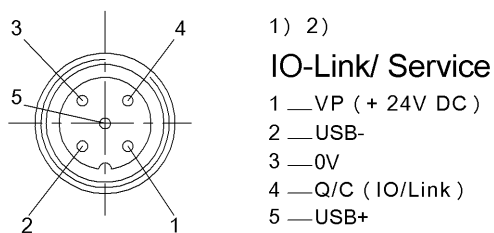
1) 視圖沿插接方向 2) 插口, 5 針 / 功能
