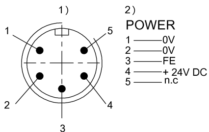
1) 視圖沿插接方向 2) 插頭, 5 針 / 功能
