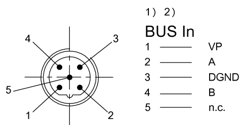
1) 視圖沿插接方向 2) 插頭, 5 針 / 功能
