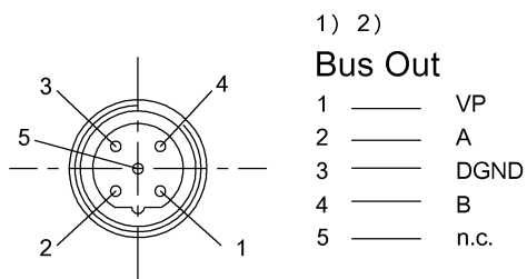
1) 視圖沿插接方向 2) 插口, 5 針 / 功能
