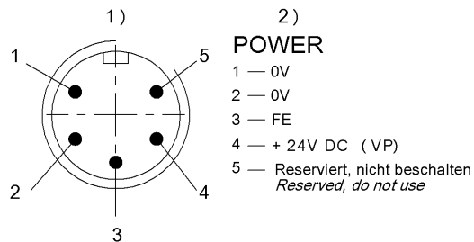
1) 視圖沿插接方向 2) 插頭, 5 針 / 功能
