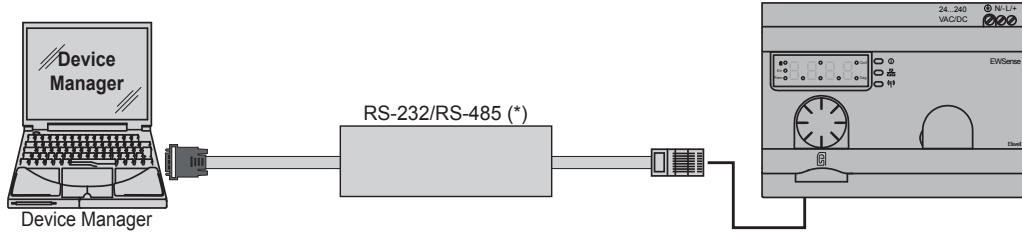
(*) RS-232/RS-485 converter / Convertitore RS-232/RS-485 / Convertidor RS-232/RS-485 / RS-232/RS-485 Wandler / Convertisseur RS-232/RS-485 / Конвертер RS-232/RS-485 / Conversor RS-232/RS-485 / محوّل التوجيه RS-232/RS-485
