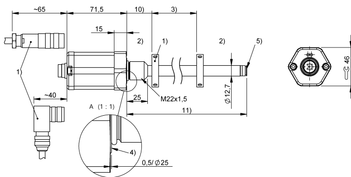
BTL7-S510-Mxxxx-CE-S32
