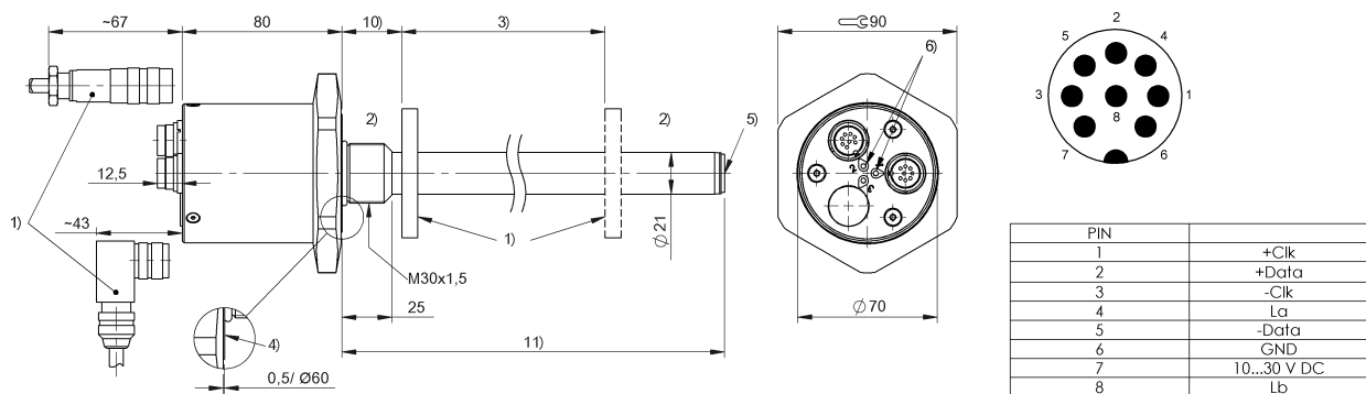
BTL7-S5xxD-Mxxxx-TT2-S32
